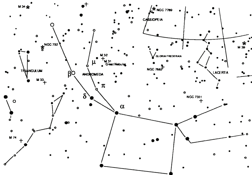
Abb. 16 Andromeda-Galaxie
