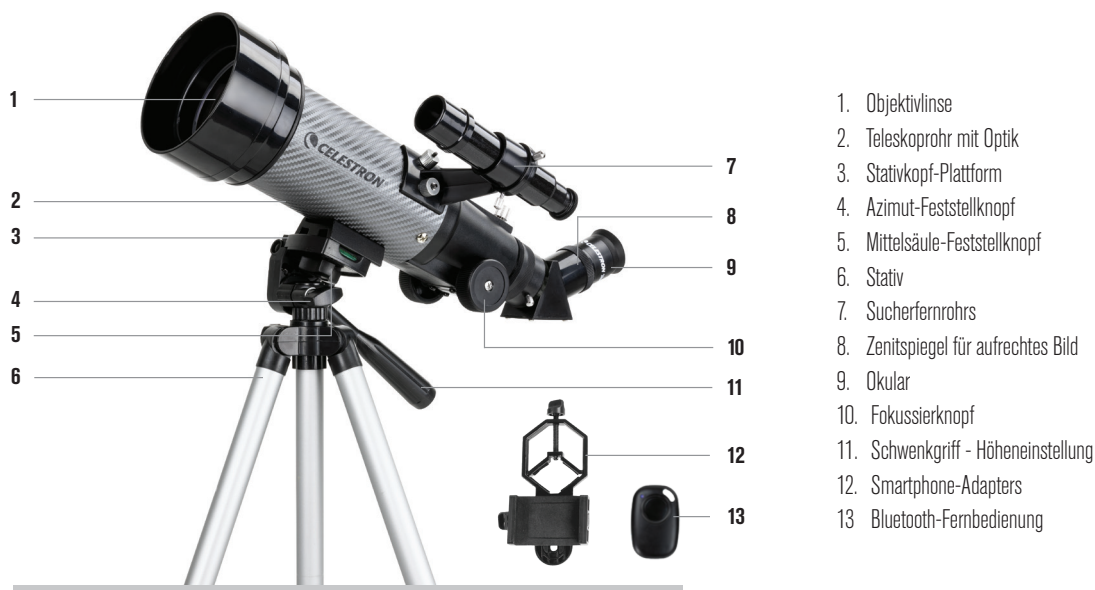
Abb. 1 Travel Scope 70DX (Travel Scope 60DX ähnlich)
